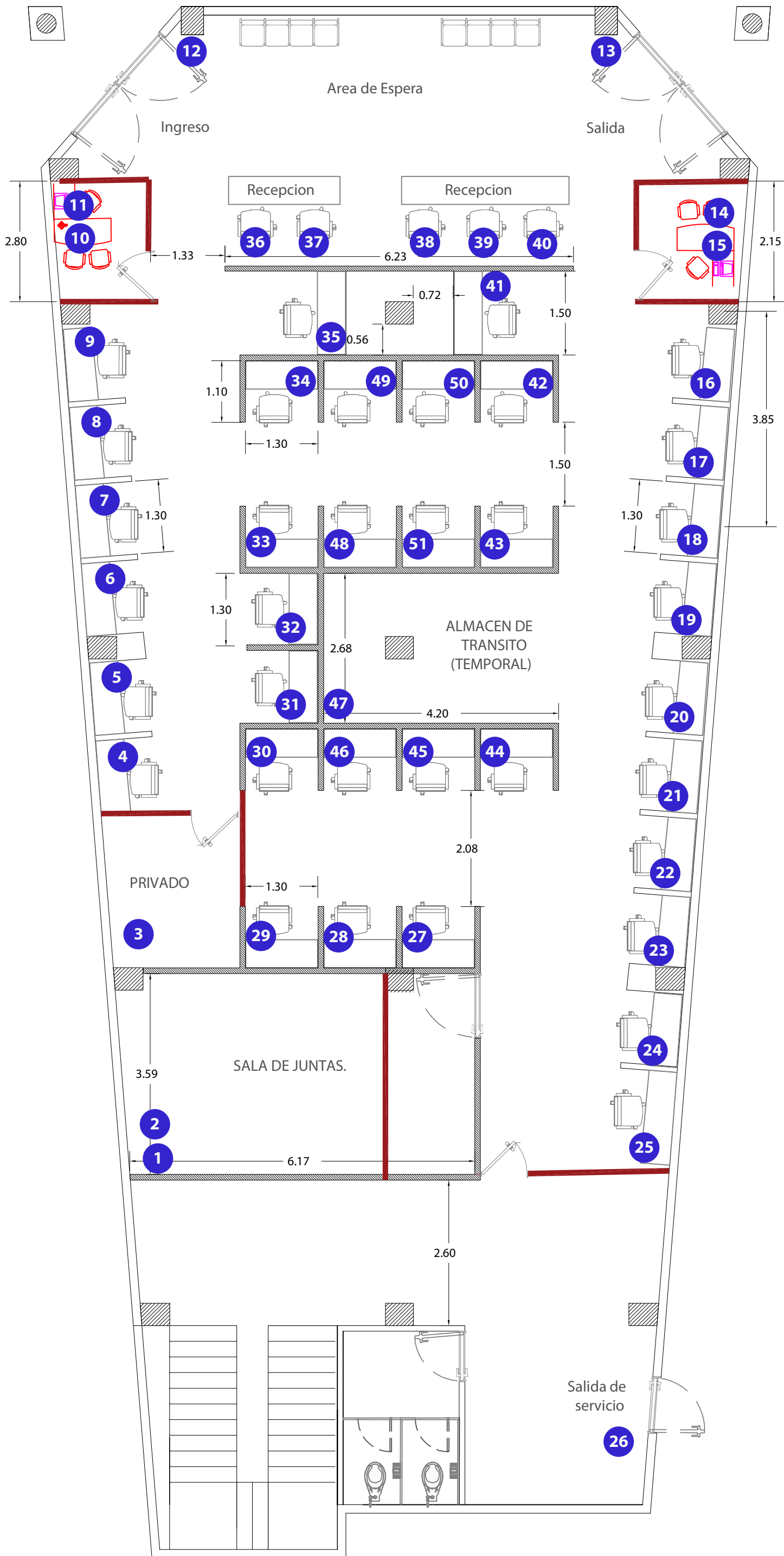
PLANTA BAJA
